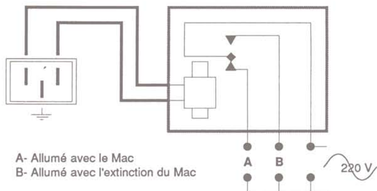
Prise arrière du Mac II
